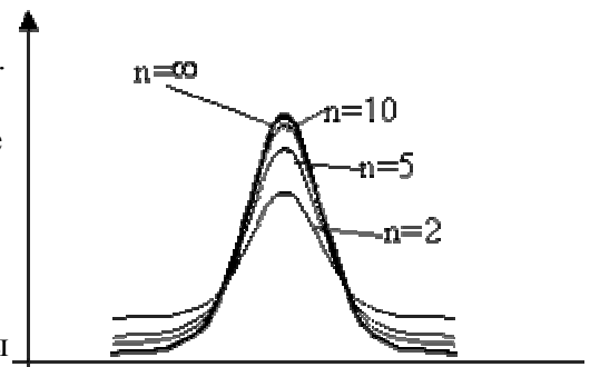
Рис. 4. Кривые Стьюдента
