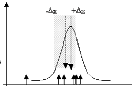
Рис. 3. Доверительный интервал
