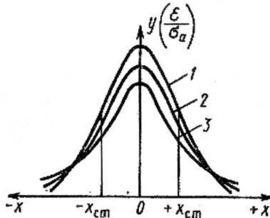
Рис.1. Кривые распределения Стюдента для различных значений:
