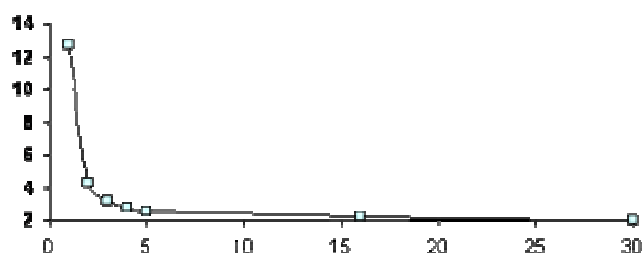
Зависимость 1 от числа ст. свободы
