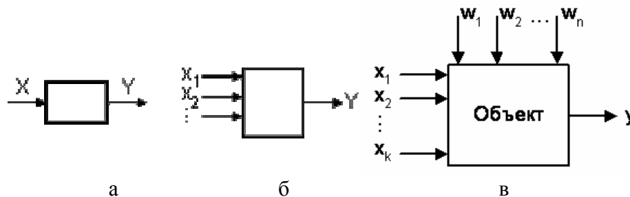
Рисунок 2. Виды экспериментов
