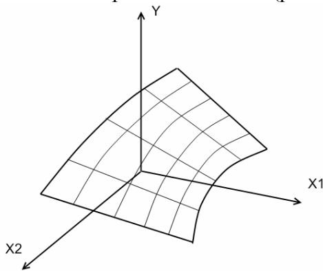
Рис. 3. Поверхность отклика
