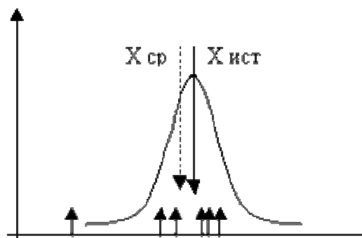
Рис. 2. Серия измерений
