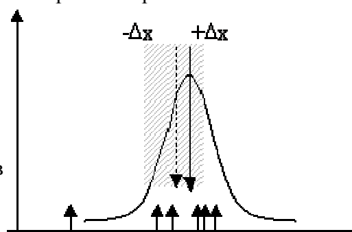
Рис. 3. Доверительный интервал
