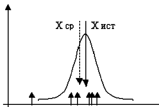
Рис. 2. Серия измерений
