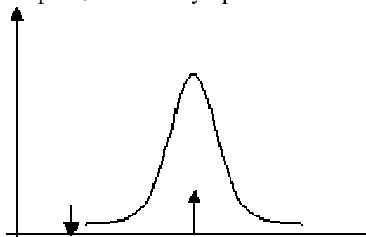
Рис. 1. Нормальное распределение
