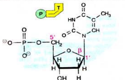
2. Дезокситимидин-5-фосфат (dTMP)
