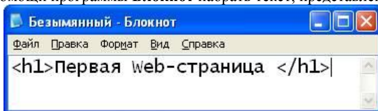
Рис. 1.3. HTML-код Web-страницы
