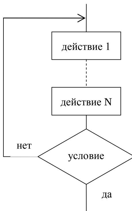
Рисунок 13 – ЦИКЛ с постусловием
