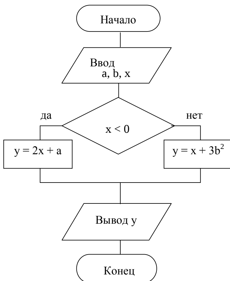
Рисунок 14 – Пример блок-схемы
