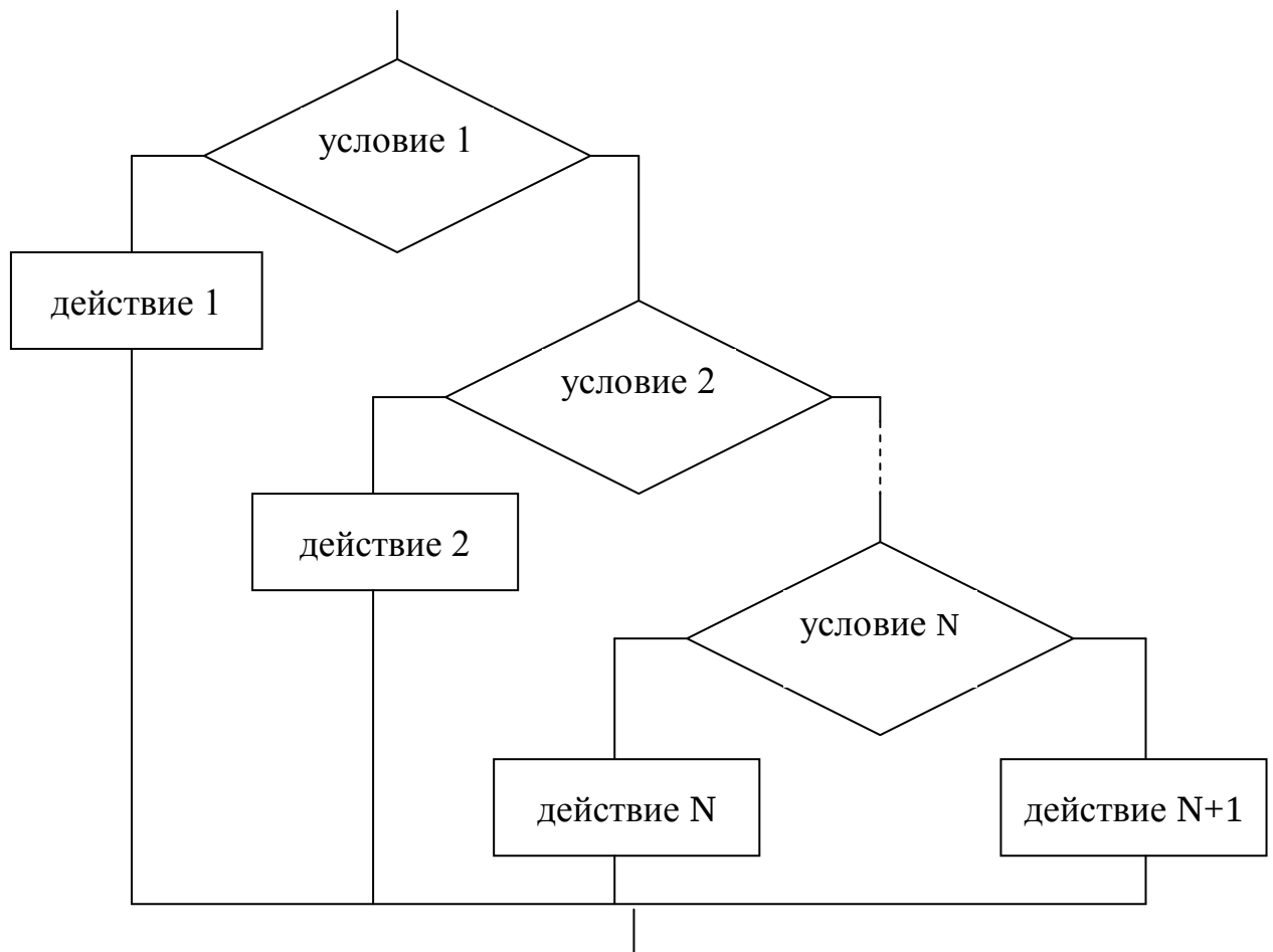
Рисунок 10 – Блок-схема ВЫБОР
