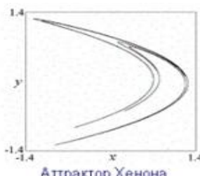
Аттрактор Хенона
