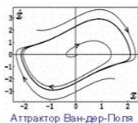
Аттрактор Ван-дер-Поля
