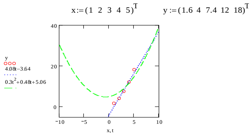
Рис. Изображение в ДСК опытных точек, линейной и квадратичной зависимостей x := (1 \ 2 \ 3 \ 4 \ 5)^T \quad y := (1.6 \ 4 \ 7.4 \ 12 \ 18)^T \text{line}(x, y) = \begin{pmatrix} -3.64 \\ 4.08 \end{pmatrix} \quad \text{или} \quad \begin{aligned} \text{intercept}(x, y) &= -3.64 \\ \text{slope}(x, y) &= 4.08 \end{aligned} f(t) := \text{line}(x, y)_0 + \text{line}(x, y)_1 \cdot t
