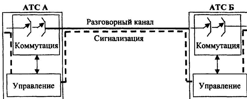
Рисунок 3 - Сигнализация по выделенному сигнальному каналу с отдельными блоками коммутации и управления
