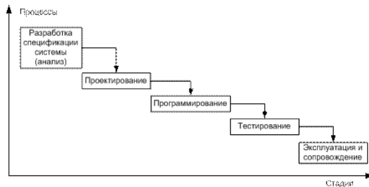
Рис.4. Каскадная модель жизненного цикла.
