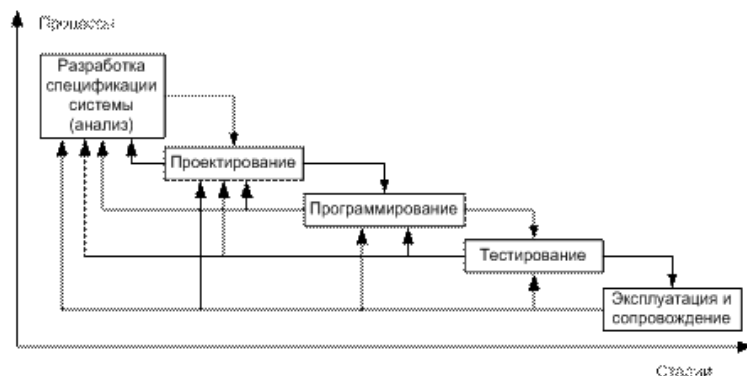
Рис.5. Модель реального процесса разработки системы.
