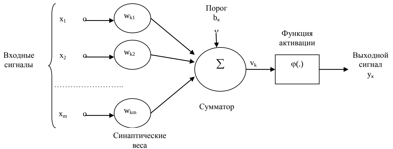
Рисунок 3 – Модель искусственного нейрона
