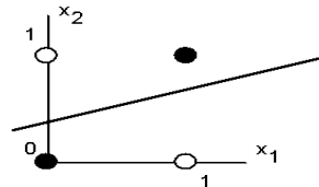
Рис. 4.2. Белые точки не могут быть отделены одной прямой от черных.
