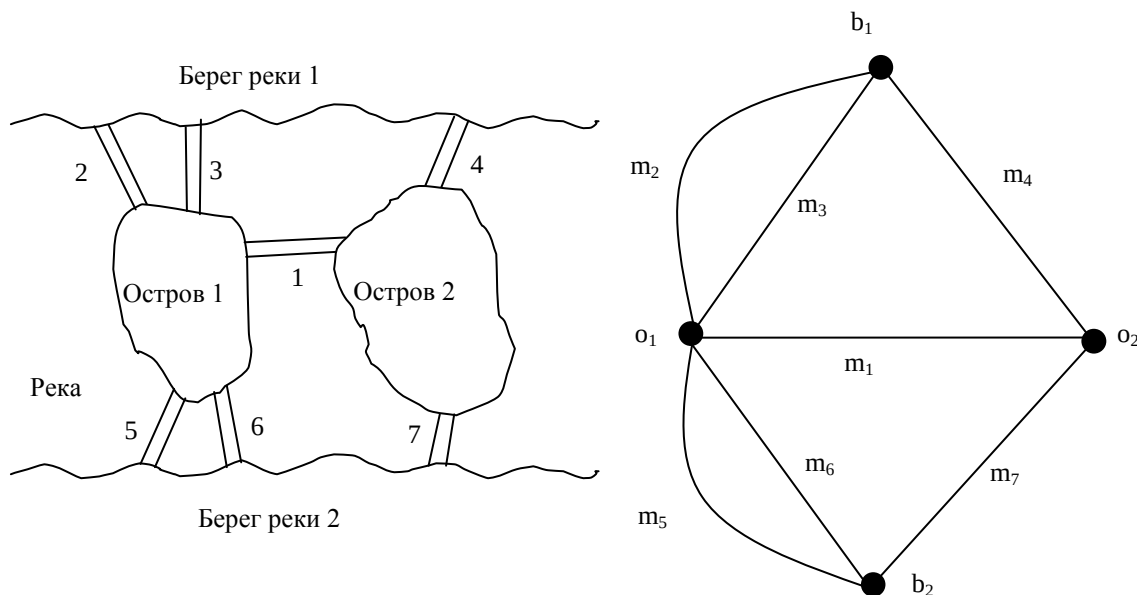
Рис.2 – Задача о кенигсбергских мостах
