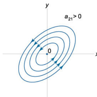
Рис. 18. Центр.
