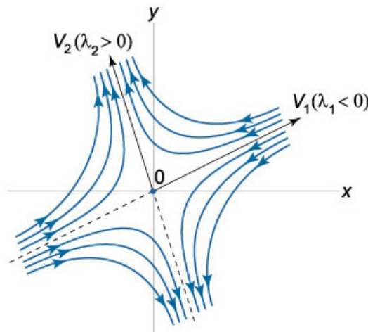
Рис. 12. Седло.
