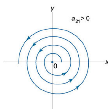
Рис. 16. Неустойчивый фокус.
