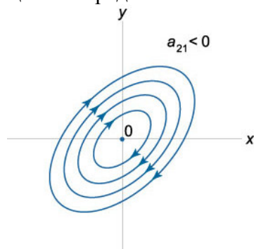
Рис. 17. Центр.
