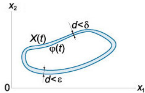
Рис. 4. Орбитальная устойчивость.
