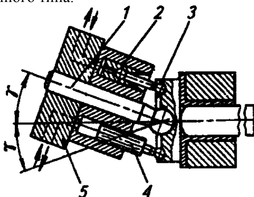
Рис. 10.6 Аксиально-поршневые насосы:
