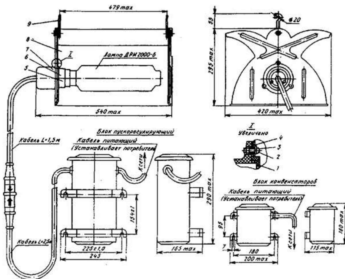
Рис. 10. Конструкция и габаритные размеры облучателя тепличного "ФОТОС-4" типа ОГС01-2000-002 У5
