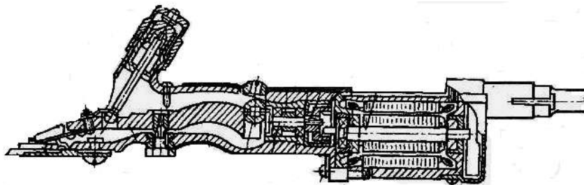
Рис. 2. Стригальная машинка MSU-200
