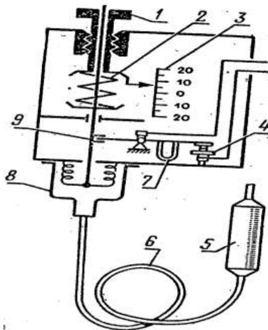
Рис. 6 Схема термореле:
