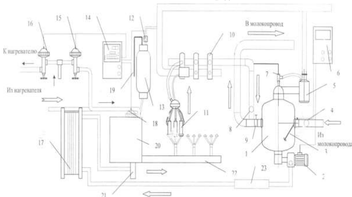
Рис. 3. Молочная 1 - молокоприемник, 2 - молочный насос, 3 - датчик уровня, 4 -- отверстие для извлечения пыжа, 5- предохранительная камера, 6 - блок управления фематроник-с, 7 - форсунка, 8 - отверстие для извлечения пыжа, 9 - заслонка, 10 - кран, 11 - доильный аппарат, 12 - кнопка заправки моющего средства, 13 - дозатор моющего средства, 14 - блок управления промывкой, 15 - кран холодной воды, 16 - кран горячей воды, 17 - пластинчатый охладитель, 18 - краны управления, 19 - шланг заправки моющего раствора, 20 - бак автомата промывки, 21 - труба слива, 22 - всасывающей трубопровод, 23 - фильтр.
