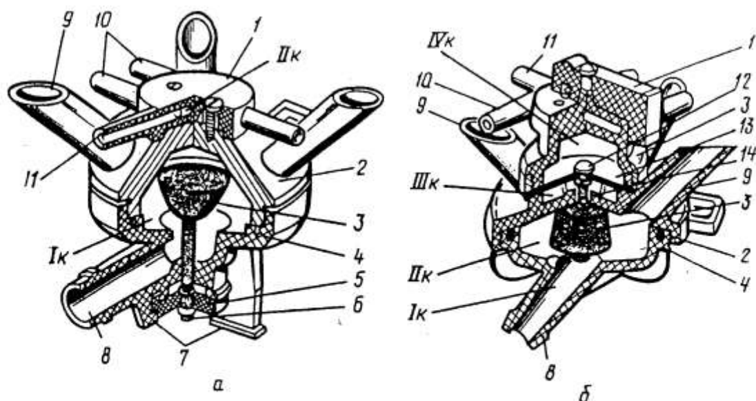
Рис. 3. Коллектор АД'У-1 двухтактной (а) и трехтактной (б) модификаций: 1 — распределитель; 2 — корпус; 3 — клапан; 4 — корпус молокосборной камеры; 5 — шайба; 6 — шплинт; 7 — выступ-фиксатор; 8 — патрубок молочного шланга; 9 — молочный патрубок; 10 — патрубок переменного вакуума; 11 — штуцер; 12 — стержень; 13 — мембрана; 14 — канал
