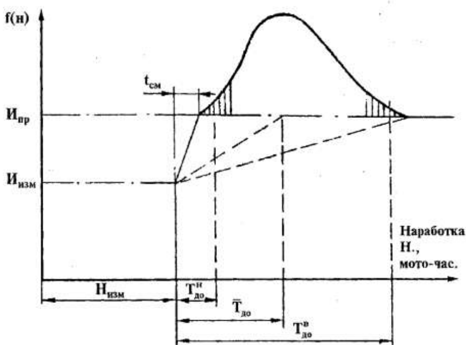
Рис. 2.2 – Схема определения доверительных границ \bar{T}_{до}
