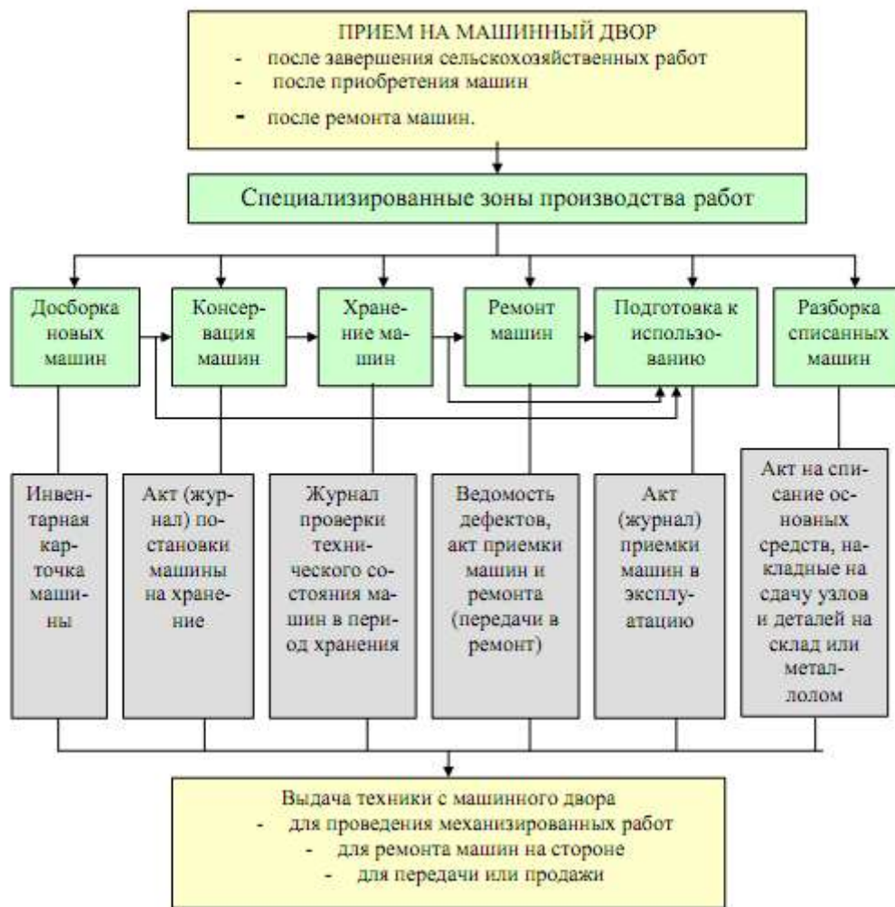
Рисунок 3 Технологическая схема проведения работ на машинном дворе
