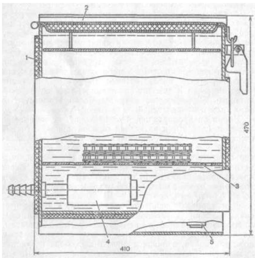
Рисунок 3. Ванна для проварки втулочно-роликовых цепей: 1 – корпус емкости; 2 – крышка; 3 – сетчатая перегородка; 4 – фильтр; 5 – сливное отверстие.
