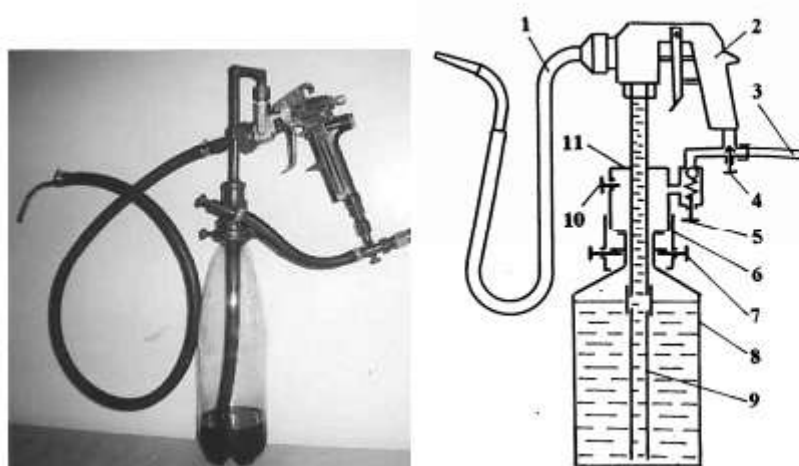
Рис. 5. Компактный аппарат ПРК-4:
