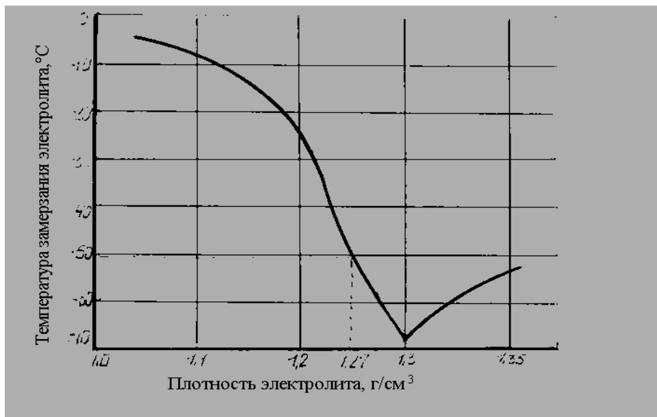
Рисунок 1 – Зависимость температуры замерзания электролита от его плотности
