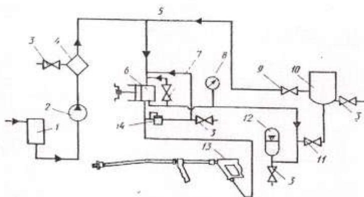
Рисунок 2 – Принципиальная гидравлическая схема очистителя ОМ-5359
