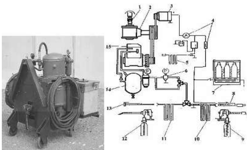
Рис. 6.8. Мобильный энергопривод МЭП-02:
