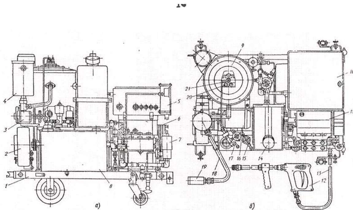
Рисунок 1 – Струйно-мониторный очиститель ОМ-5359
