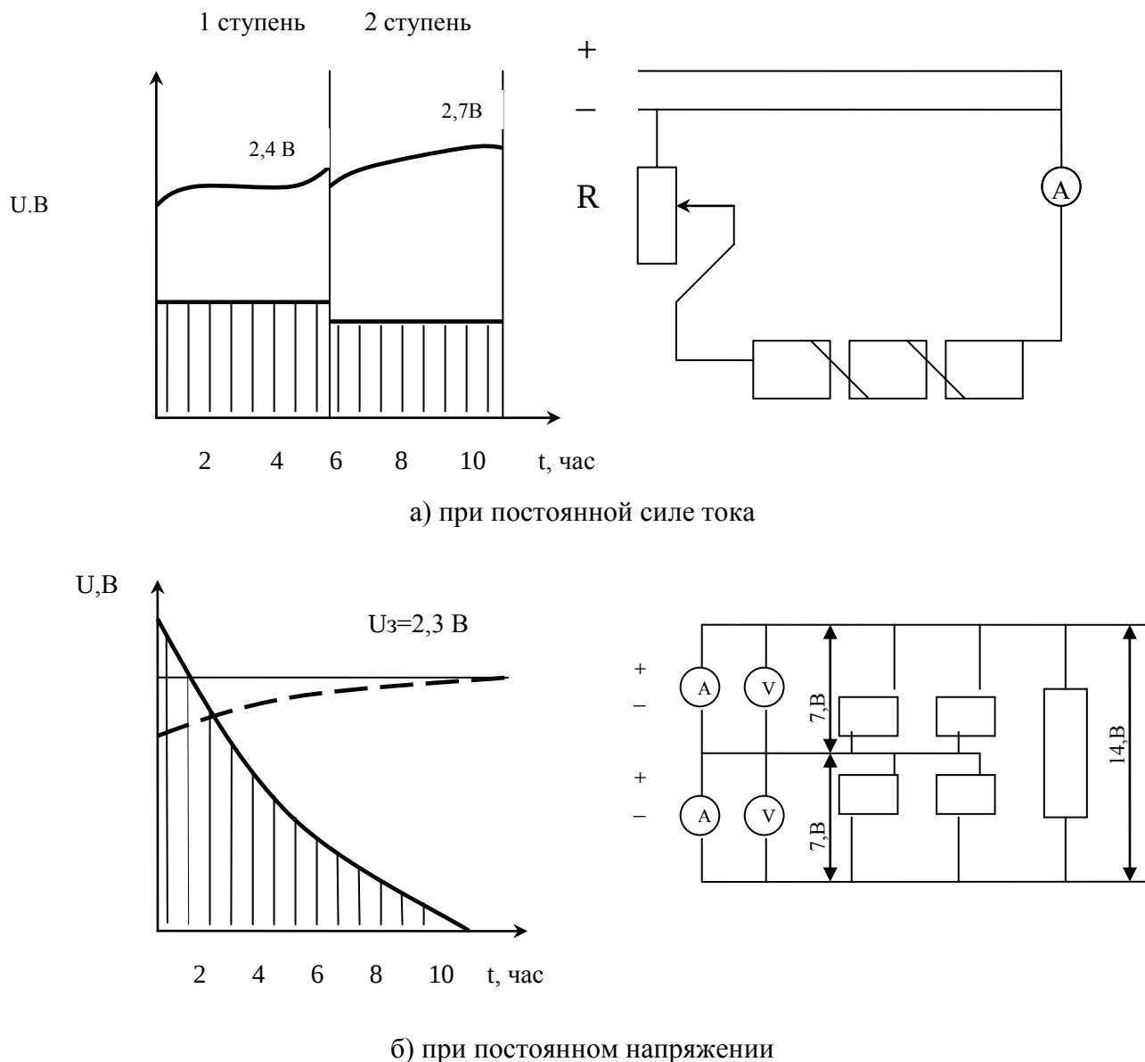
Рисунок 1 - Методы зарядки аккумуляторных батарей
