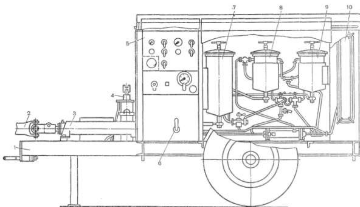
Рисунок 2. Универсальный передвижной агрегат для подготовки техники к хранению: 1 – шасси полуприцепа 1-ПТС-2; 2 – карданный вал; 3 – промежуточный вал; 4 – гидроподъемник; 5 – пульт управления; 6 – рычаг включения масляного насоса; 7 – емкость жидкого консервационного материала (лакокрасочных материалов); 8 – емкость защитной смазки; 9 – емкость противокоррозионной присадки; 10 – шланги выдачи консервационных составов.
