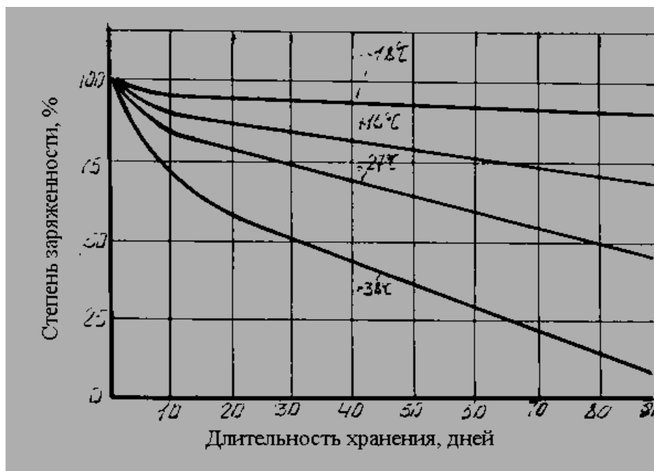
Рисунок 2 – Характеристика саморазряда аккумуляторной батареи в зависимости от температуры и длительности хранения (в днях)
