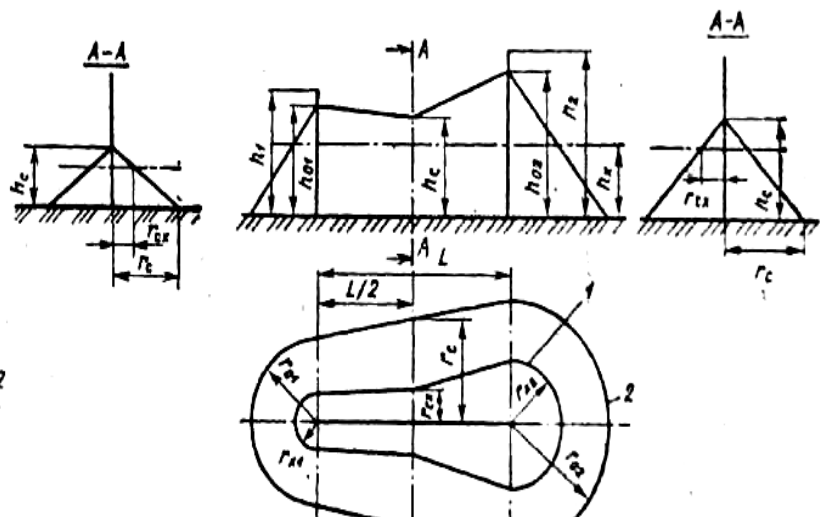
Рис. 3. Зона защиты двойного стержневого молниеотвода разной высоты.
