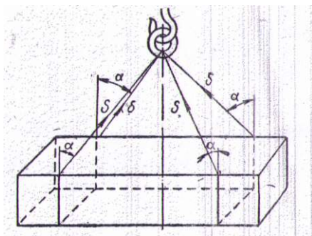
Рис. 1. Схема к расчету чалок.
