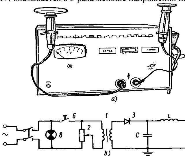
Рис. 17. Электрический дефибриллятор: а - общий вид; б - упрощенная принципиальная схема. 1 - повышающий трансформатор 127 (220)/6000 В; 2 - регулятор напряжения; 3 - диод; 4 - электроды; 5 - грудная клетка пострадавшего; 6 - кнопка заряда; 7 - кнопка разряда; 8 - сигнальная лампа; L - индуктивное сопротивление 0,3 Гн; C - конденсатор 20 - 25 мкФ. У современных дефибрилляторов оба электрода одинаковые и представляют собой металлические
