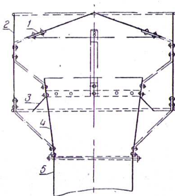
Рис. 2. Дифлектор ЦАГИ
