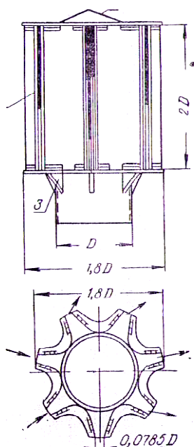
Рис. 3. Звездообразный дефлектор:
