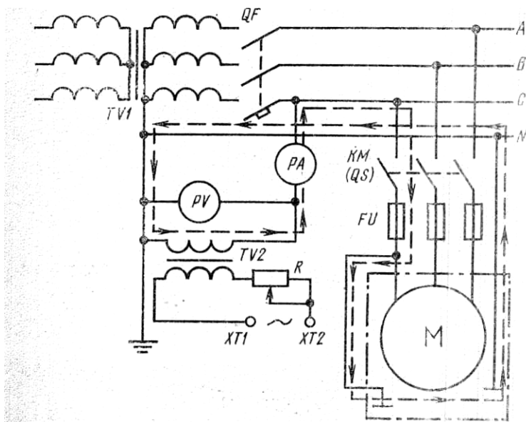
Рис. 1. Схема измерения сопротивления петли проводников «фаза - нуль» по методу амперметра и вольтметра
