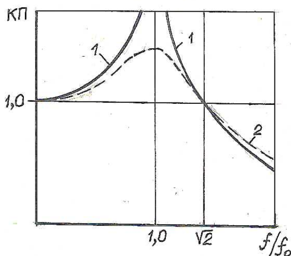
Рис.6.1. Зависимость коэффициента передачи (КП) от частоты возмущающей силы: 1 – без учета затухания колебаний в амортизаторах; 2 – с учетом затухания.
