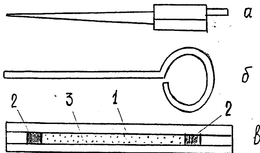
Рисунок 2 - Принадлежности для снаряжения индикаторной трубки: а - стержень, б - штырь, в - снаряженная индикаторная трубка, 1 - стеклянная трубка, 2 – ватный пыж, 3 – индикаторный порошок.
