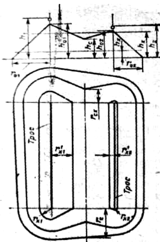
Рис. 6. Зона защиты двух тросовых молниеотводов разной высоты.
