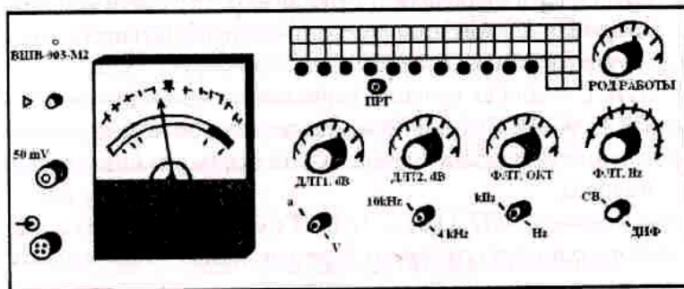
Рис. 4. Измеритель шума и вибрации ВШВ-003-М2 (лицевая панель)
