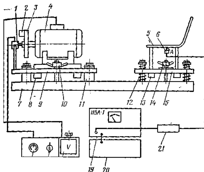
Рис 1. Схема установки для исследования вибраций:
