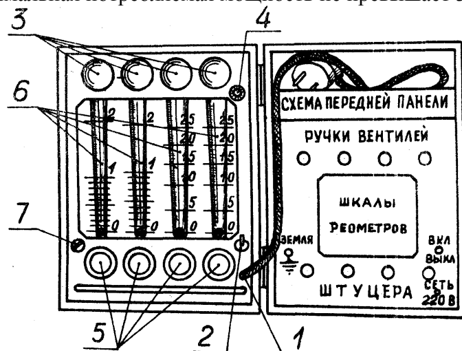
Рисунок 2 - Схема общего вида ротационной установки ПРУ-4 для отбора проб воздуха
