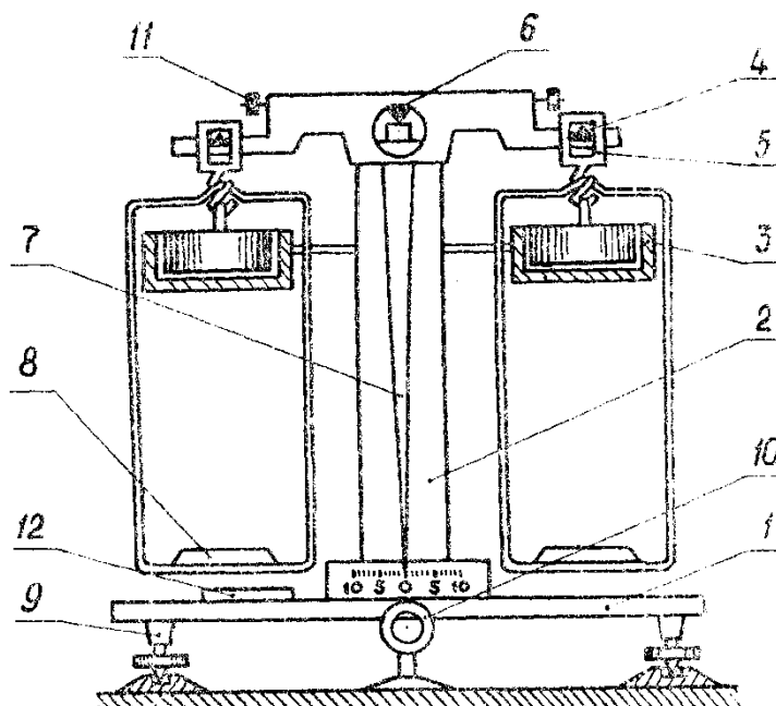
Рисунок 3 - Схема аналитических весов типа ВЛА-200
