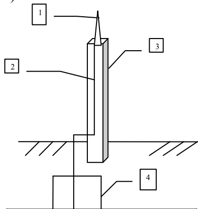
Рис. 3 Схема устройства молниеотвода
