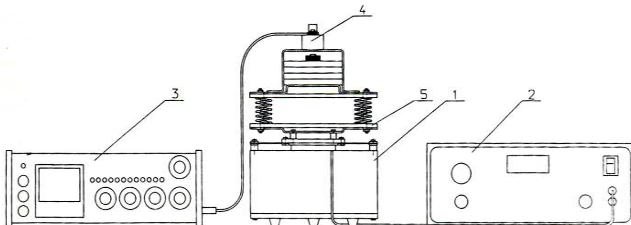
Рис.2. Установка «Вибростенд»
