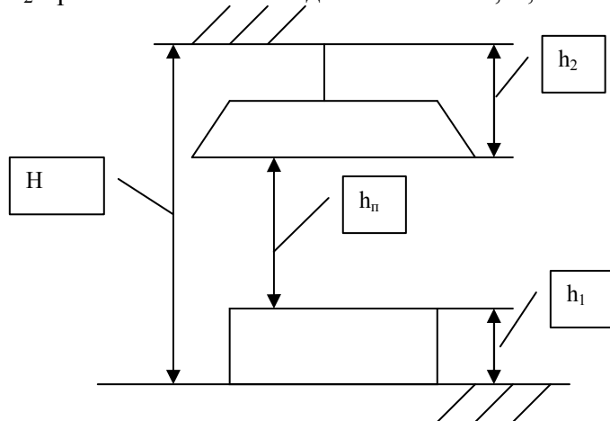
Рис. 2 Схема подвеса светильника над рабочим местом
