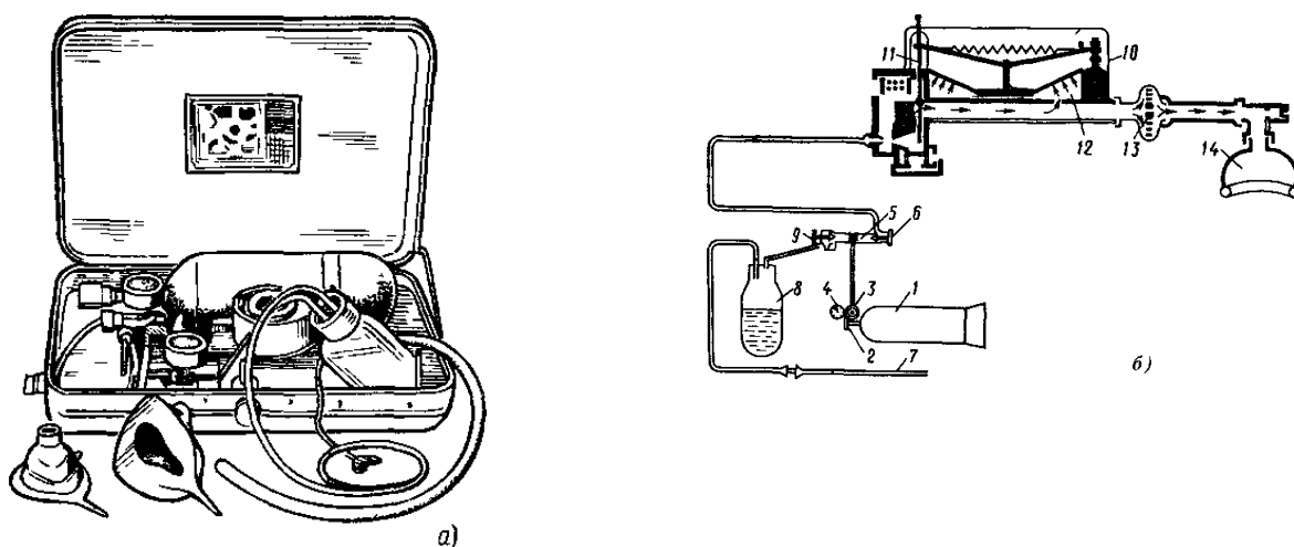
Рис 8. Аппарат ДП-2 для длительного искусственного дыхания с активным вдохом и выдохом а - общий вид б - принципиальная схема (при положении «вдох»)
