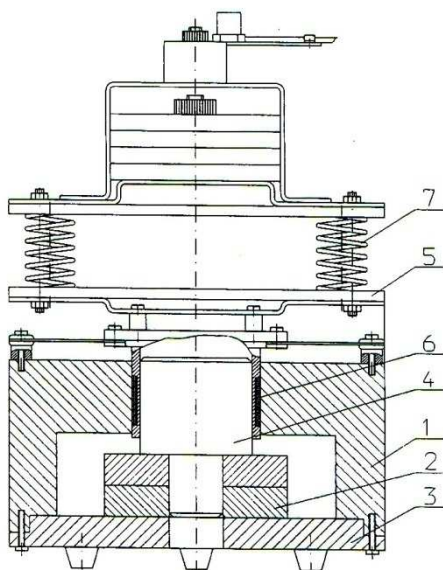
Рис.2. Установка «Вибростенд»
