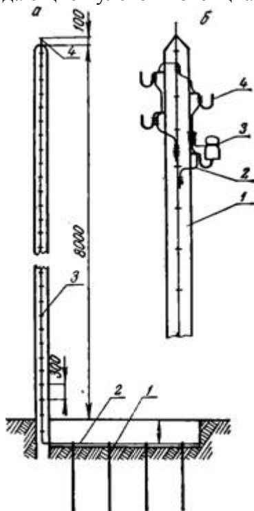
Рис. 9. Заземляющее устройство на деревянной опоре: а — общий вид, б — заземление крюков
