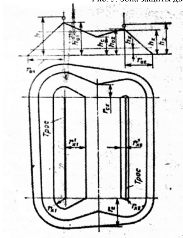
Рис. 5. Зона защиты двойного тросового молниеотвода.
