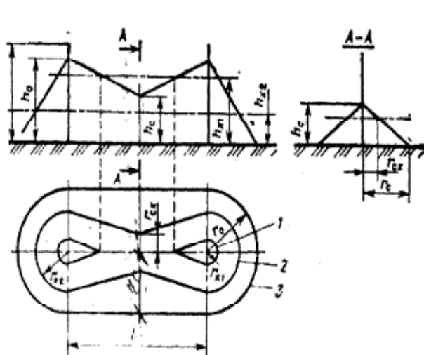
Рис. 2. Зона защиты двойного стержневого молниеотвода
