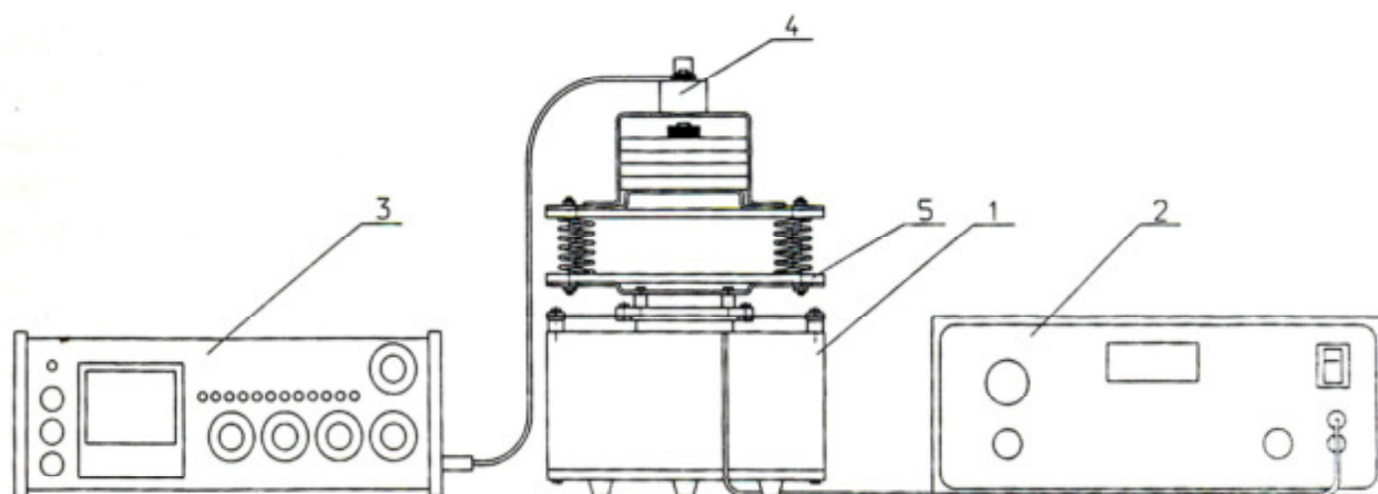
Рис.2. Установка «Вибростенд»
