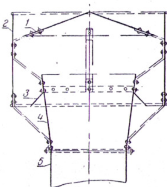
Рис. 2. Диффлектор ЦАГИ
