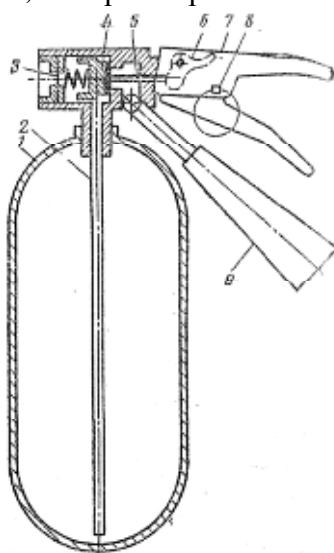
Рис.1 Схема огнетушителя ОХВП-10:
