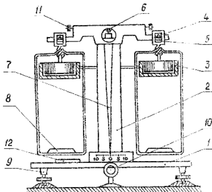
Рисунок 3 - Схема аналитических весов типа ВЛА-200
