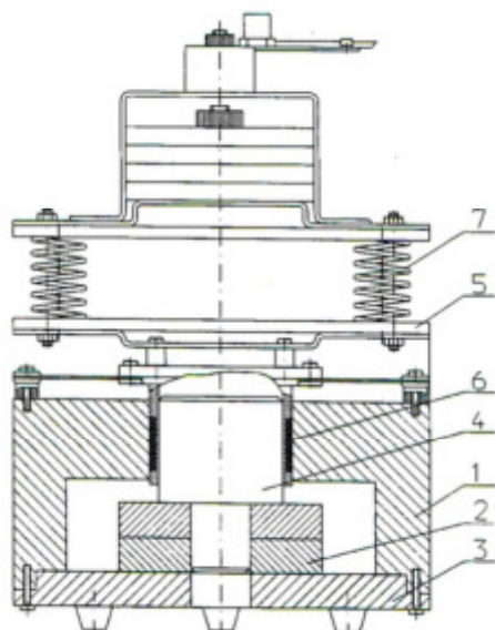
Рис.2. Установка «Вибростенд»
