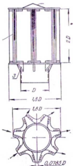
Рис. 3. Звездообразный дефлектор:
