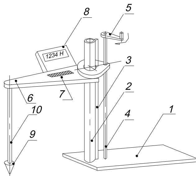
Рис. 3. Тензометрический твердомер.
