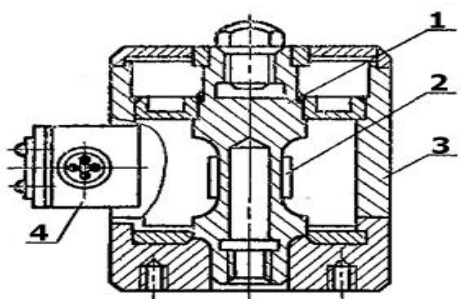
Рисунок 1 -Конструкция тензодатчика
