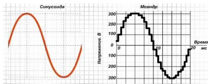
Рис.5 – Форма выходного напряжения сетевого инвертора (синусоида)
