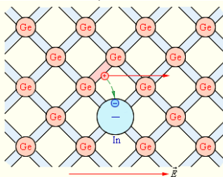
Рис. 3 - Атом индия в решетке германия. Полупроводник p – типа.
