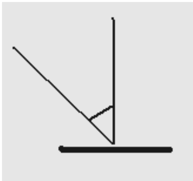
Рис. 1 Наклонное падение света
