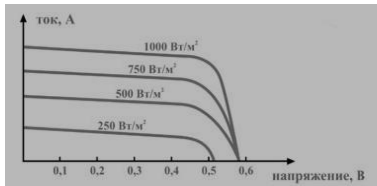
Рис.6 - Семейство нагрузочных характеристик кремниевого фотопреобразователя при различной освещённости.
