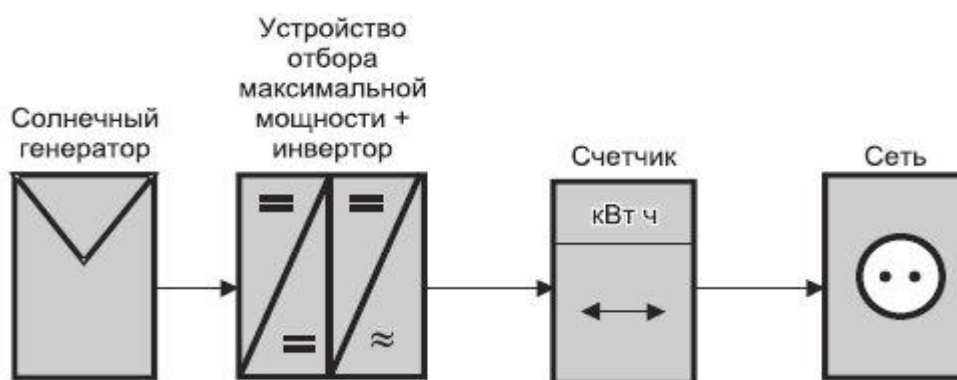
Рис. 1 - Структурная схема типовой сетевой солнечной электростанции (верхний рисунок) или в упрощённом виде (на нижнем рисунке).
