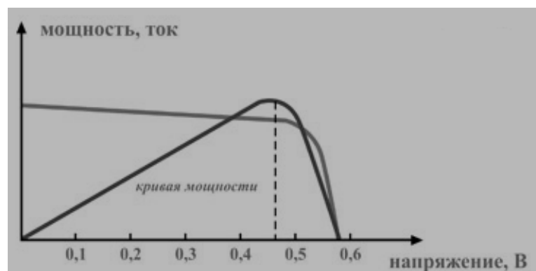
Рис.7 – График зависимости выходной мощности от напряжения для фотопреобразователя из кристаллического кремния.
