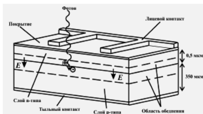
Рис. 4 - Схема кремниевого монокристаллического солнечного элемента (ФЭП).
