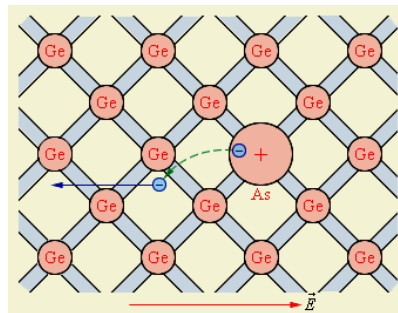
Рис.2 – Атом мышьяка в решетке германия. Полупроводник n-типа.
