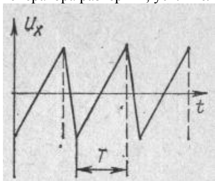
Рис.5 – График зависимости напряжения сигнала генератора развёртки, от времени
