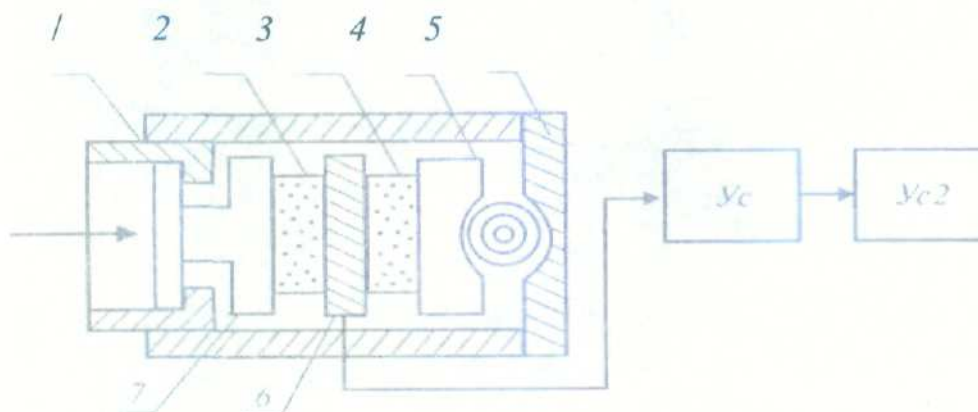
Рис. 9. Пьезометрический манометр
