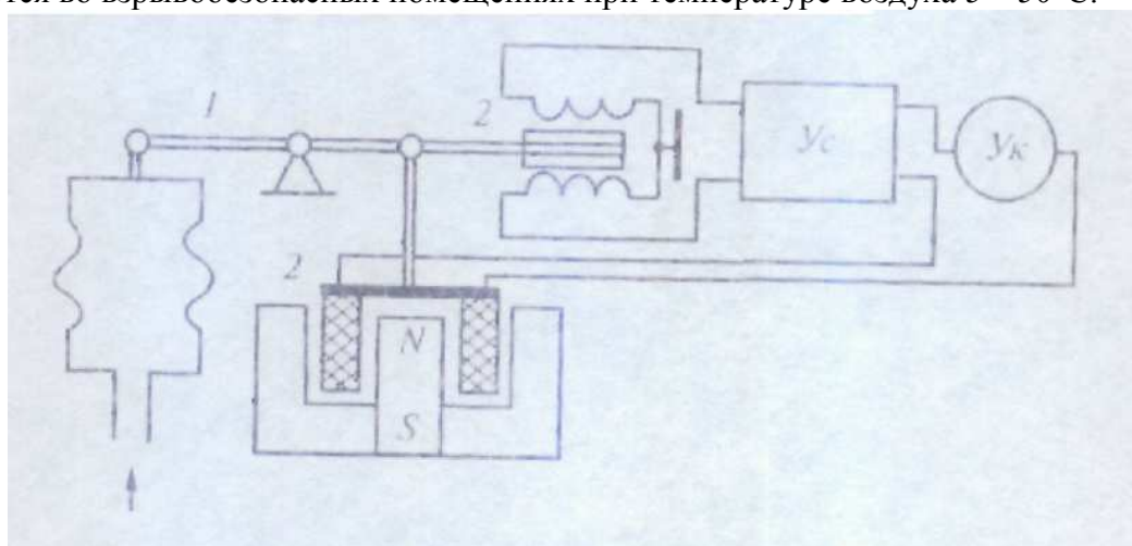
Рис. 8. Манометр уравнивающего преобразования с силовой компенсацией.
