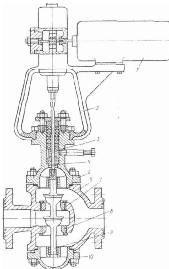
Рис. 3. Устройство регулирующего клапана:
