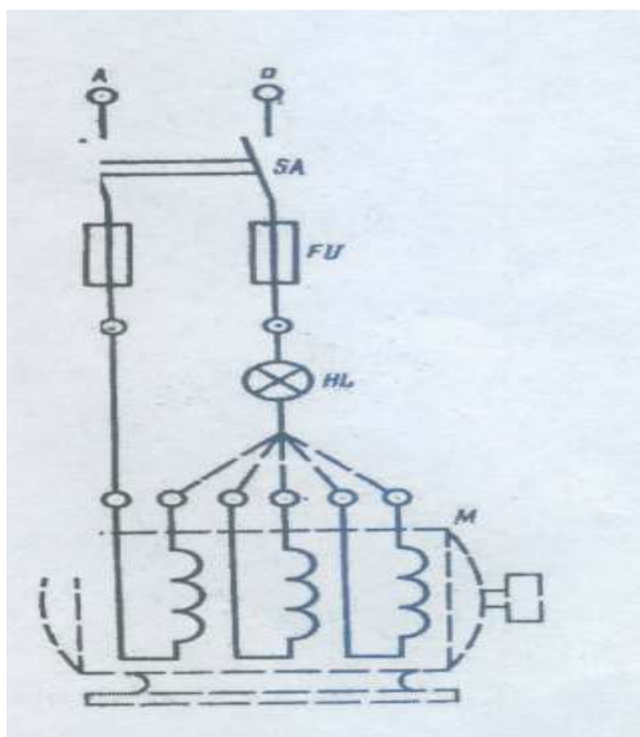
Схема определения выводов обмотки электродвигателя
