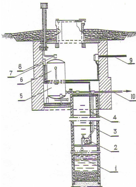
Рис. 20. Схема безбашенной водоканки:
