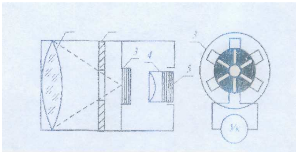
Рис. 5. Радиационный пирометр.
