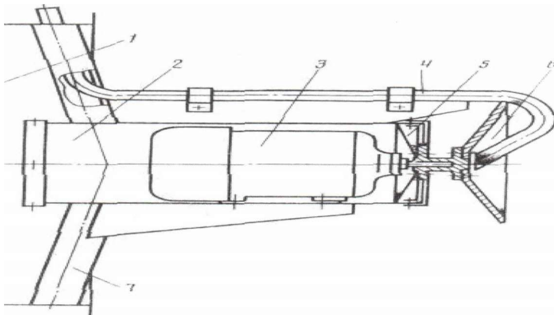
Рис. 2. Устройство разбрызгивателя: 1 — конфузор; 2—каркас; 3— электродвигатель; 4—трубка; 5— крыльчатка; 6—диск; 7 — трубчатые стойки.
