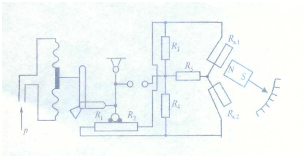
Рис. 6. Электромеханический
