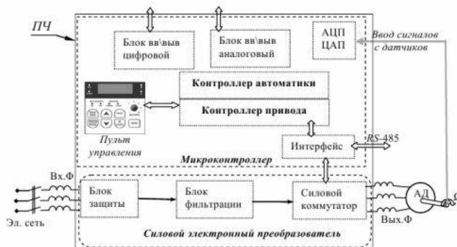
Рис. 3. Типовая структура управления асинхронным двигателем с использованием преобразователя частоты
