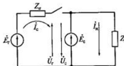
Рис. 1. Схема включения трехфазного синхронного генератора на параллельную работу с сетью (ламповый синхроскоп включен при этом на потухание света)
