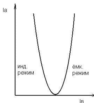
Рис. 4 U-образная характеристика синхронного компенсатора
