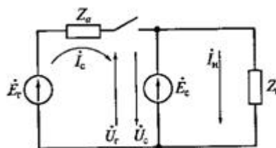
Рис. 1. Схема включения трехфазного синхронного генератора на параллельную работу с сетью (ламповый синхроскоп включен при этом на потухание света)
