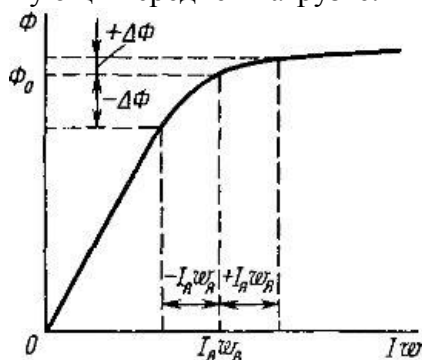
Рис. 6. Влияние степени намагничивания на результирующий магнитный поток ( I_b \cdot w_b — м.д.с обмотки возбуждения; I_a \cdot w_a — м.д.с обмотки якоря).
