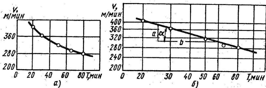
Рис.3 . Зависимость между скоростью резания и стойкостью:
