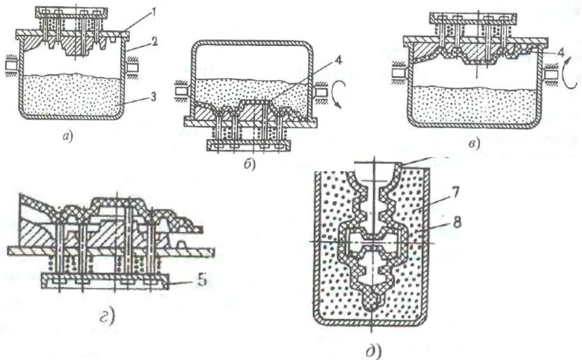
Рис. 1. Схема литья в оболочковой форме
