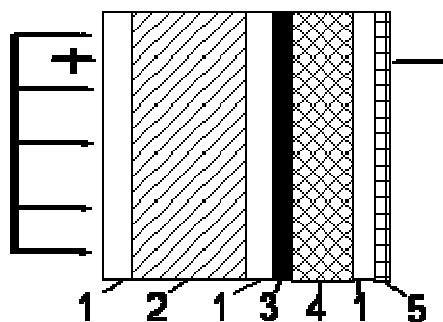
Рис. 1 – Строительно-изоляционная конструкция внутренней стены мясорыбной камеры: 1 – штукатурка, \delta = 20 мм, \lambda = 0,9 Вт/м×град; 2 – кирпичная кладка, \delta = 120 мм, \lambda = 0,7 Вт/м×град; 3 – пароизоляция (битум), \delta = 4 мм, \lambda = 0,18 Вт/м град; 4 – теплоизоляция (пенополистирол), \lambda = 0,04 Вт/м град; 5 – отделочный слой (плитка), \delta = 5 мм, \lambda = 2,2 Вт/м×град.
