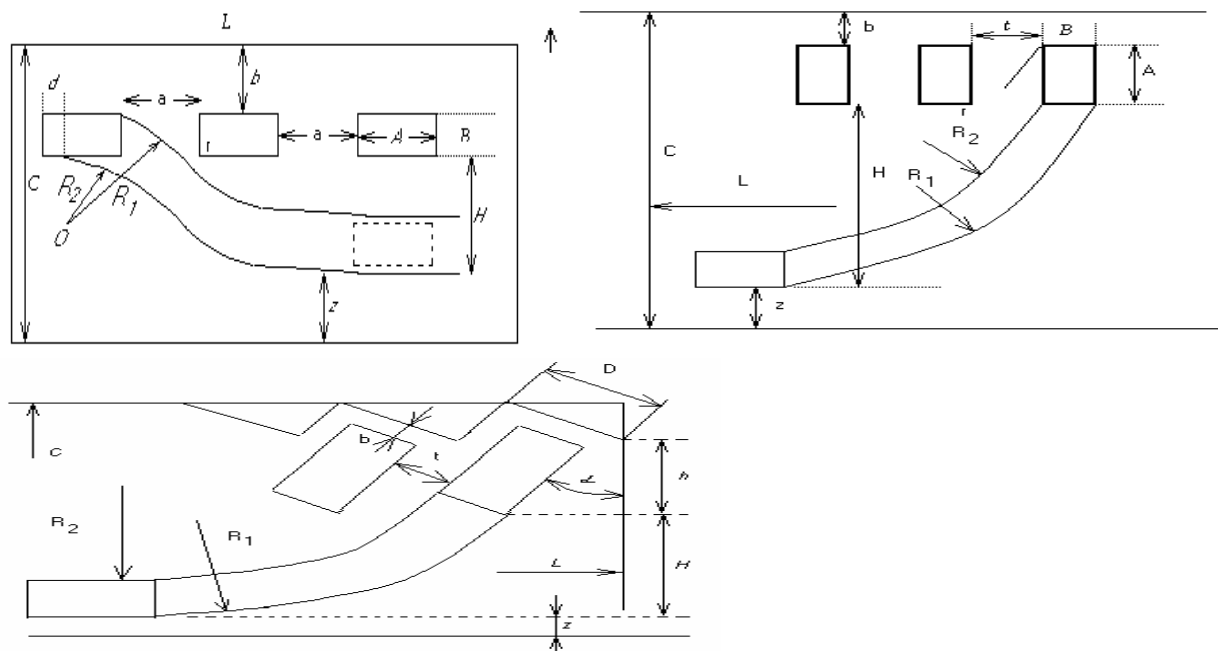
Рисунок 1 - Схемы для расчета площадки для маневрирования при различных способах расстановки автотранспортного средства: a — поточная (боковая); b — торцевая; в — ступенчатая
