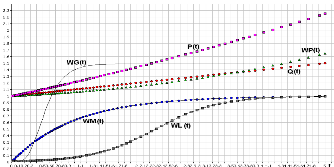
Рис.2.8. Функции роста:
