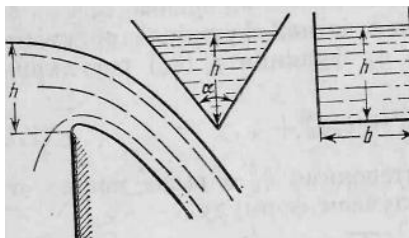
Рис. 2. Перетекание тяжелой жидкости через водослив.
