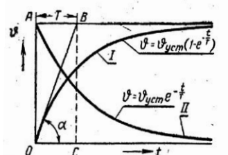
Рис. 68. Кривые нагрева и охлаждения двигателя: I — кривая нагрева; II — кривая охлаждения.
