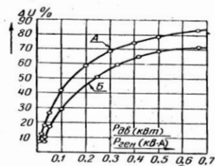
Рис. 143. Кривые потери напряжения в процентах при прямом пуске асинхронных двигателей от синхронных генераторов: а — работающих холостую; б — работающих с 50% индуктивной нагрузки.
