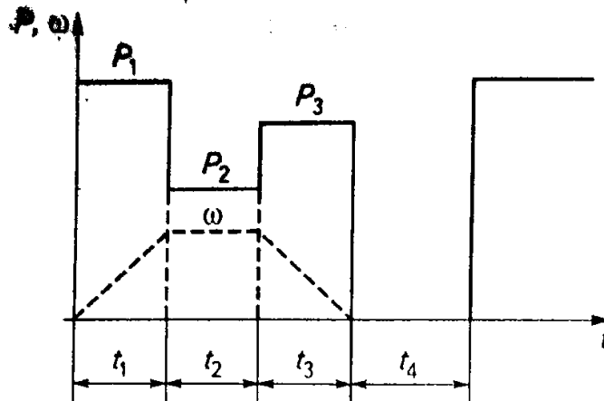
Рис. 9 Нагрузочная диаграмма.
