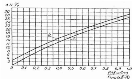
Рис. 142. Кривые потери напряжения в процентах при прямом пуске асинхронных двигателей от силовых трансформаторов: а — работающих холостую; б — работающих с 50% индуктивной нагрузки.
