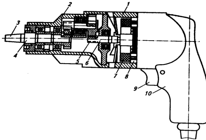
Рис. 3 Конструкция электродрели:
