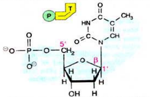
2. Дезокситимидин-5-фосфат (dTMP)
