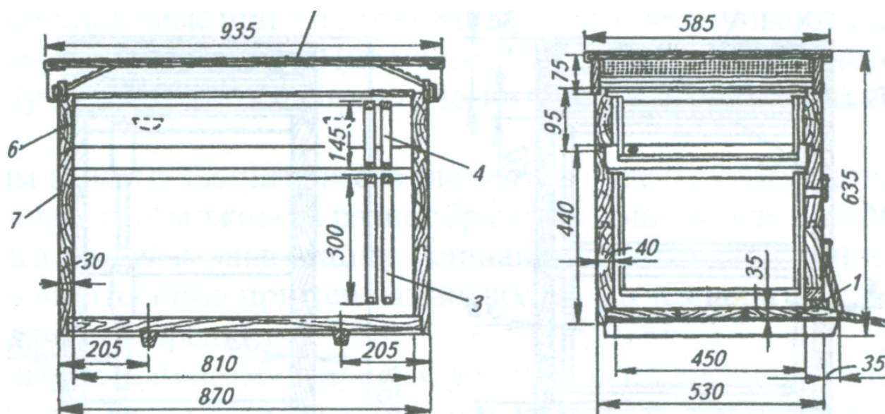
Рис. 6 Улей лежак
