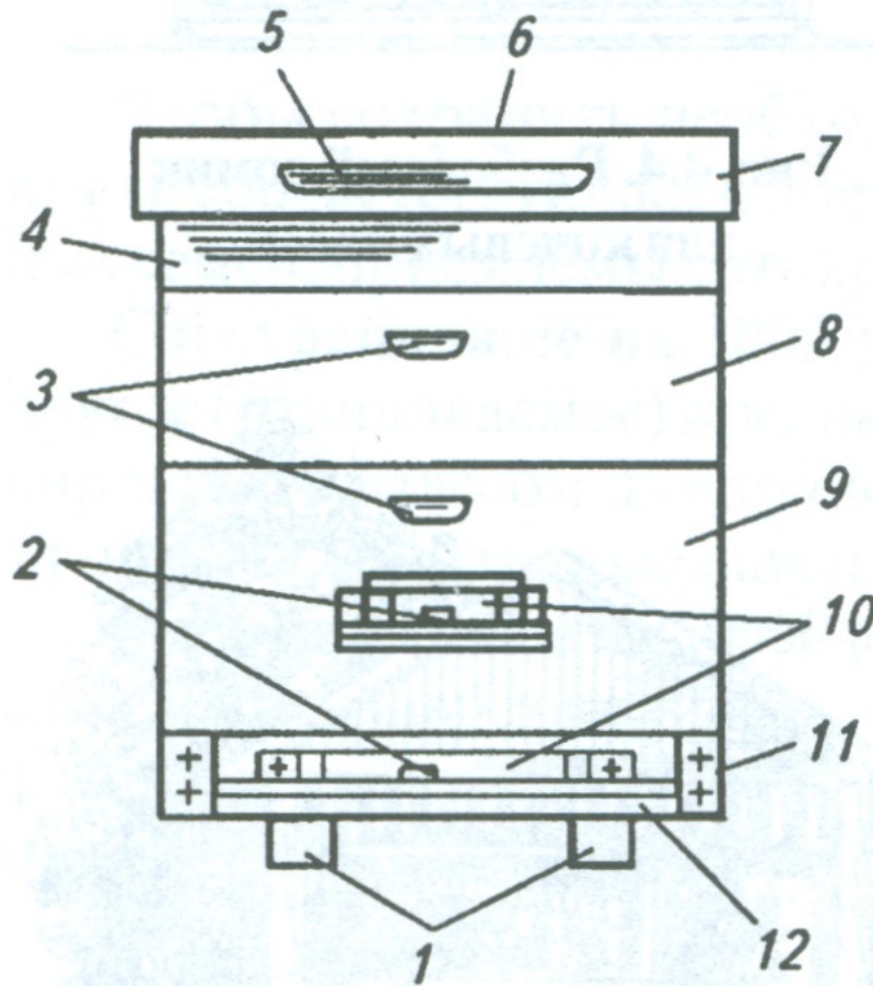
Рис. 2 Устройство улья:
