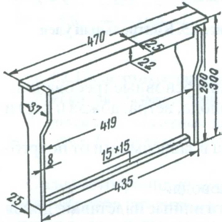
Рис.3 Гнездовая рамка
