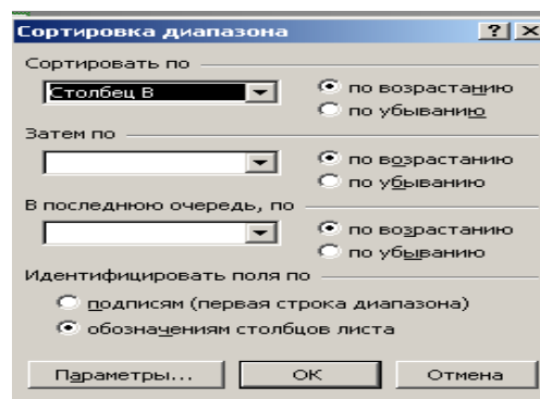
Рисунок 6 – Сортировка данных
