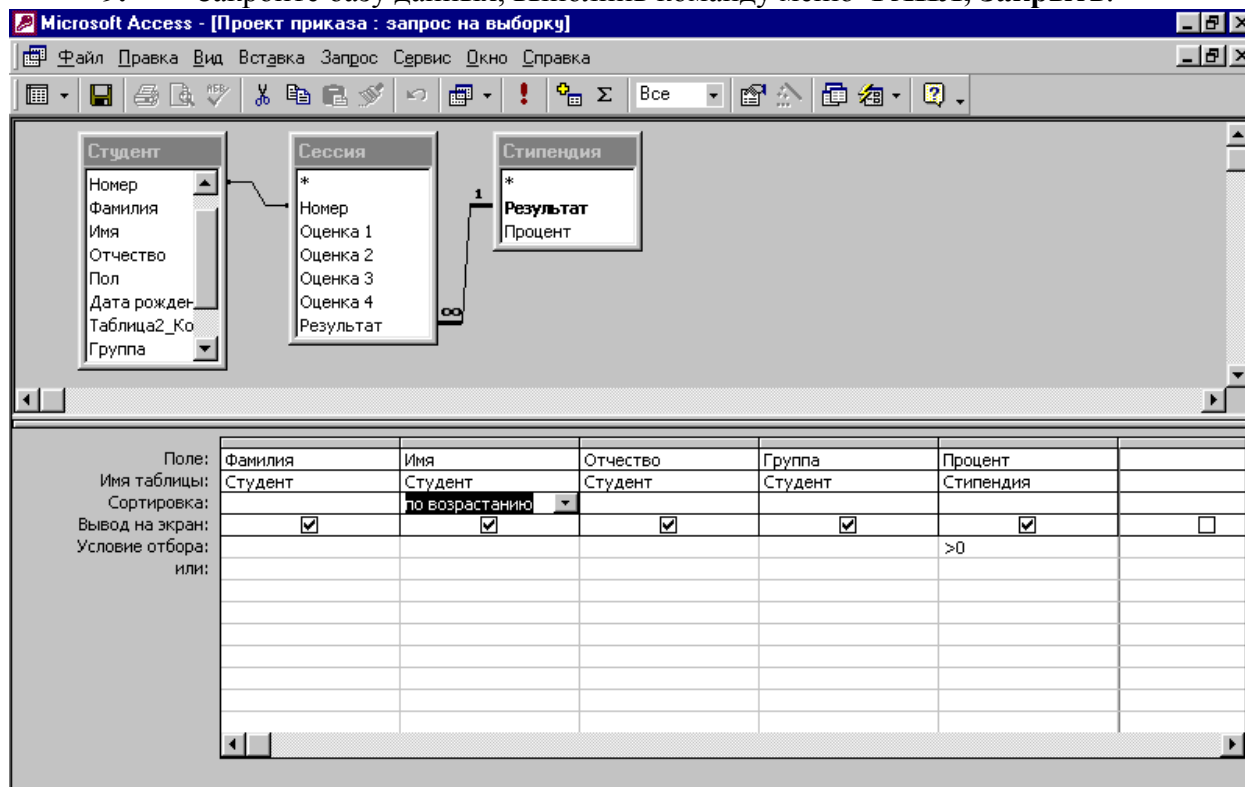
Рис.9. Окно конструктора запроса
