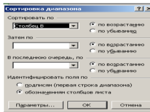
Рисунок 6 – Сортировка данных
