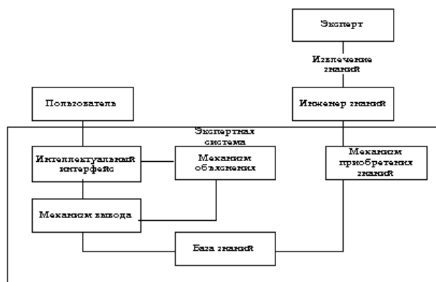
Рис. 2. Архитектура ЭС
