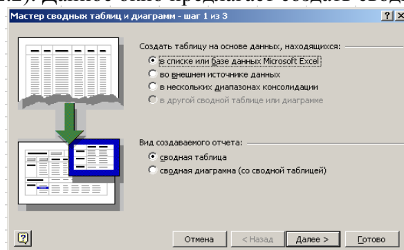
Рисунок 2.2 – Диалоговое окно Мастера сводных таблиц
