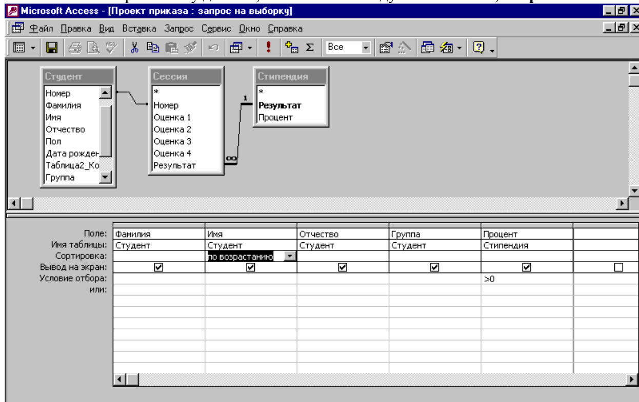
Рис.9. Окно конструктора запроса
