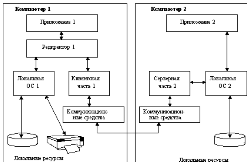
Рисунок 38. взаимодействие компонентов операционной системы при взаимодействии компьютеров
