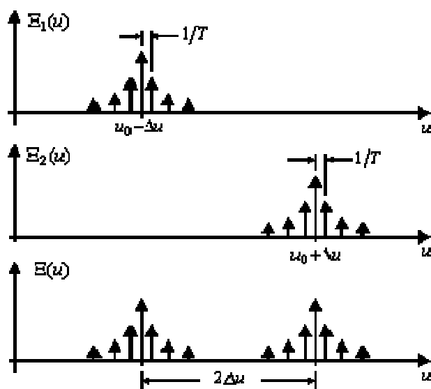
Рис. 13. Спектры частотно манипулированного сигнала
