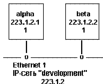
Рисунок 4 - Одна физическая сеть
