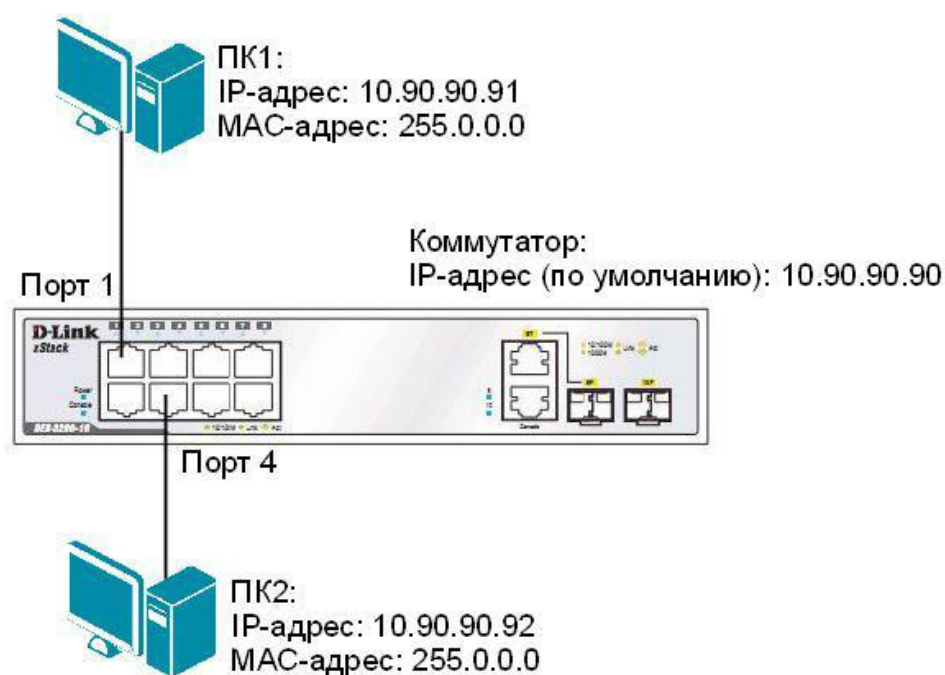
Рисунок 1.1 Схема сети
