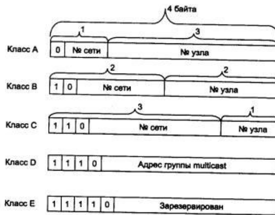
Рисунок 1 - Структура IP-адреса
