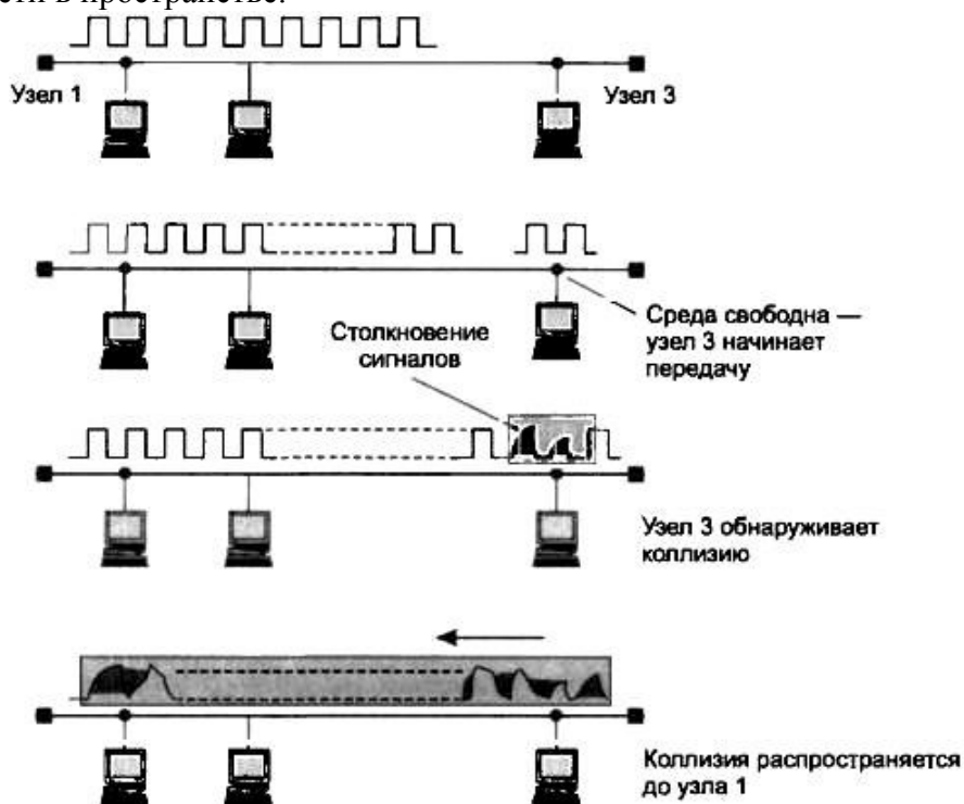
Рисунок 28 Схема возникновения и распространения коллизии
