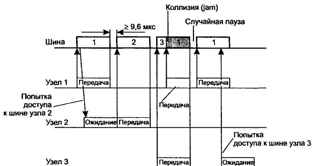
Рисунок 27 – Метод случайного доступа CSMA/CD
