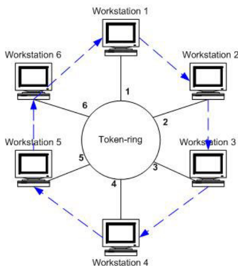
Рисунок 42 - Топология TokenRing
