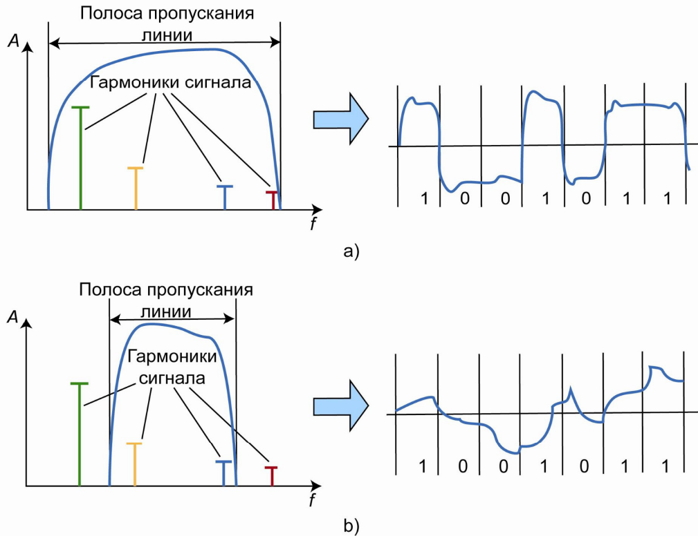
Рис. 2. Влияние полосы пропускания на сигнал
