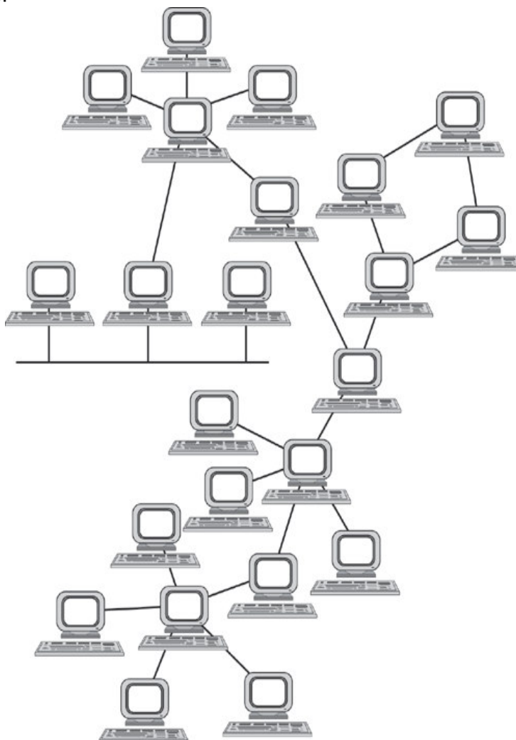
Рисунок 8 - Смешанная топология
