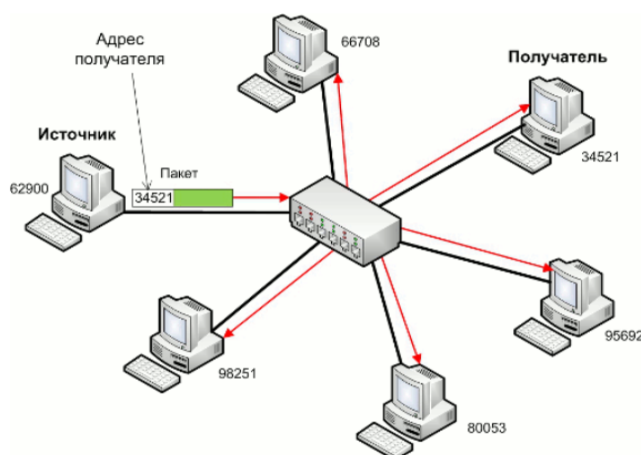
Рисунок 17. Пример работы сети с концентратором
