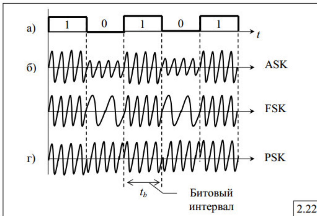
Рисунок 33. Дискретная модуляция
