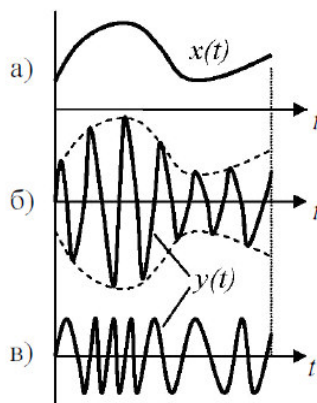
Рисунок 30. Аналоговая модуляция
