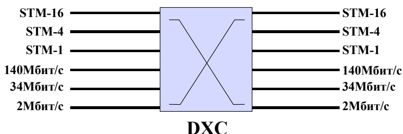
Рисунок 47. SDH кросс-коннектор
