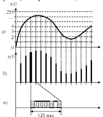
Рисунок 31. АИМ
