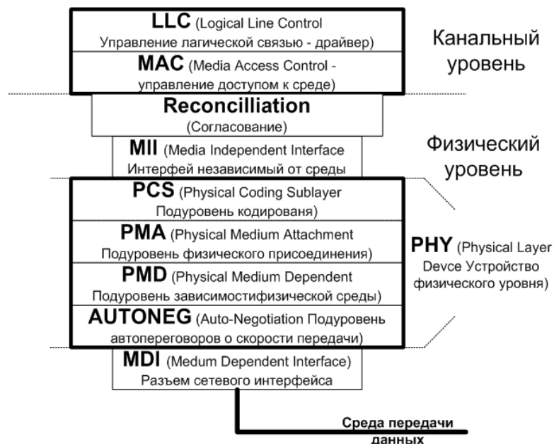
Рисунок 29. Система Fast Ethernet
