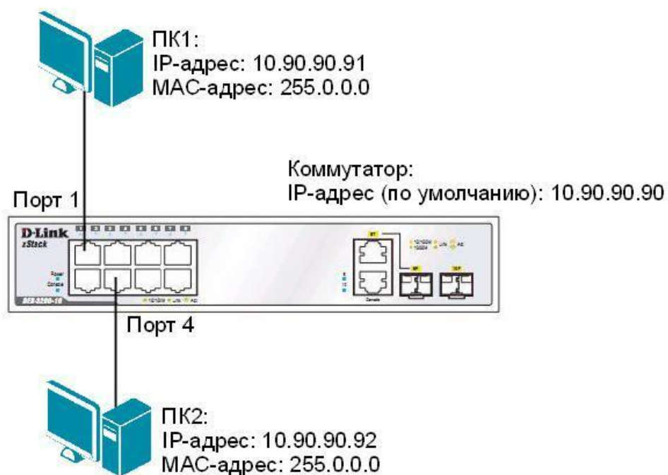
Рисунок 1.1 Схема сети
