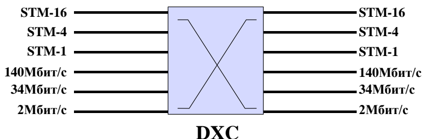
Рисунок 47. SDH кросс-коннектор
