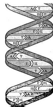
Рис. 1. Участок двуспиральной молекулы ДНК
