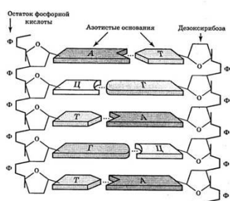
Рис. 2. Схематическое изображение молекулы ДНК
