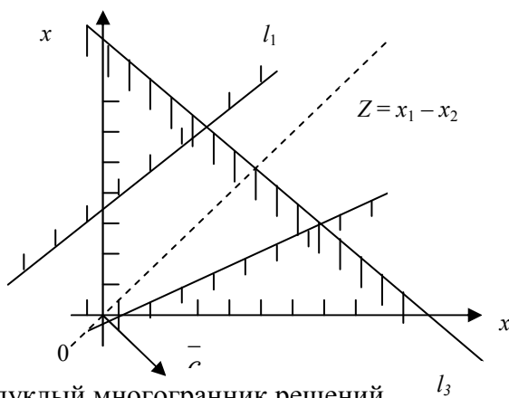
Рисунок 3 – Выпуклый многогранник решений
