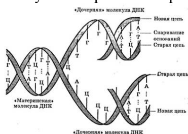
Рис. 4 Репликация ДНК
