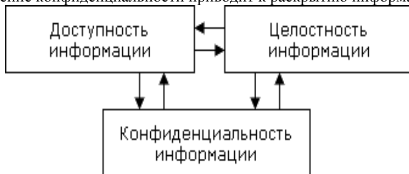
Рисунок Составляющие информационной безопасности
