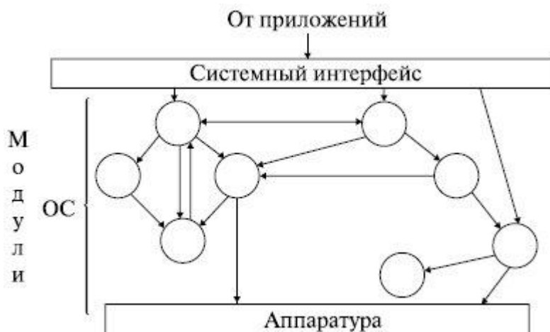
Рис. 1.2. Монолитная архитектура
